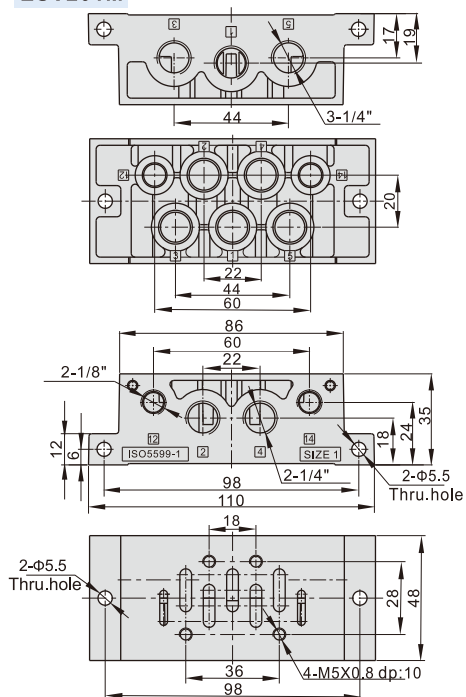
ESV201M
