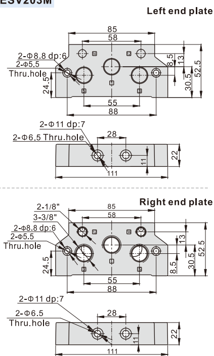
ESV203M
