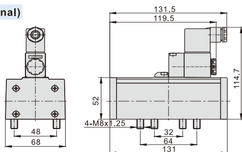
ESV410 (Grommet)
