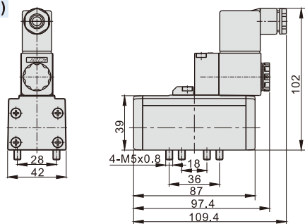
ESV210 (Terminal)
