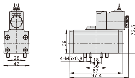
ESV220(Grommet)
