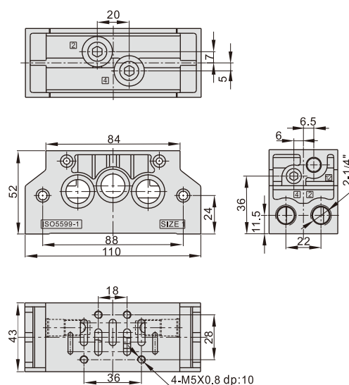
ESV202M
