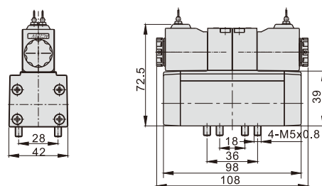
ESV230(Grommet)
