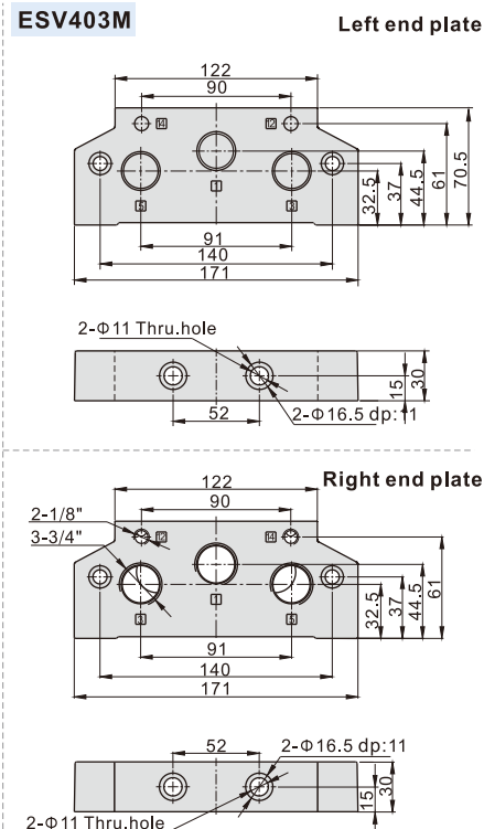
ESV403M
