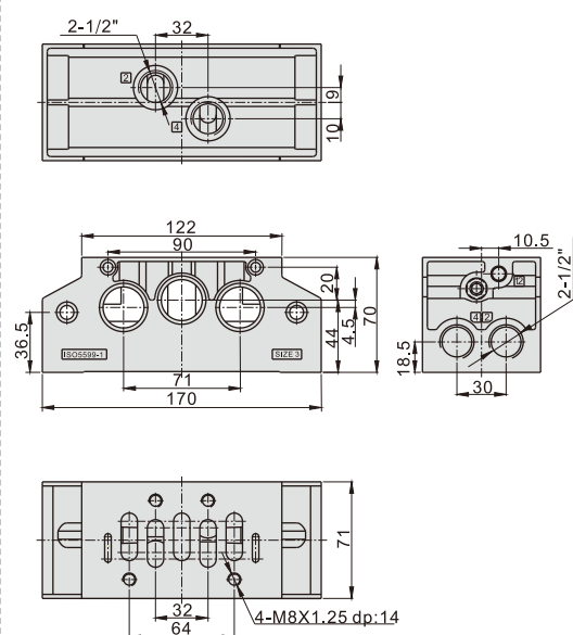
ESV402M
