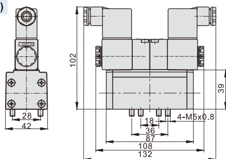
ESV220(Terminal)
