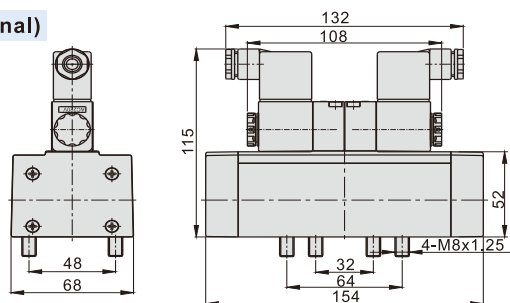
ESV402M
